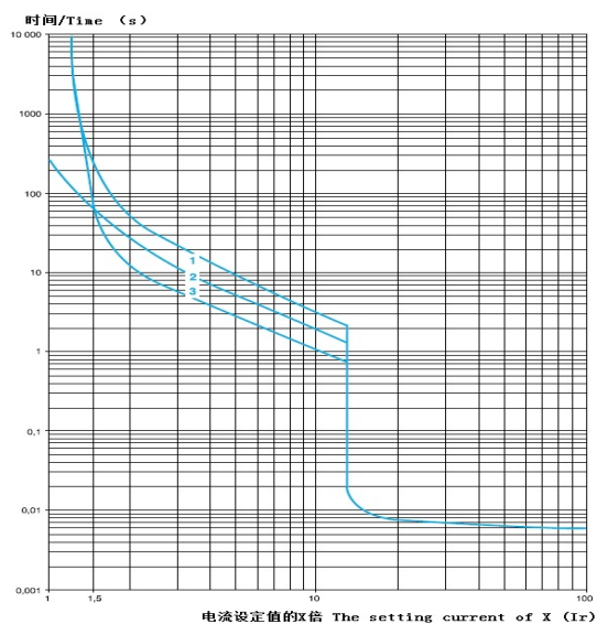
NDD1-32 电流时间特性曲线 20±2℃/NDD1-32 current/time characteristic curve 20±2℃
